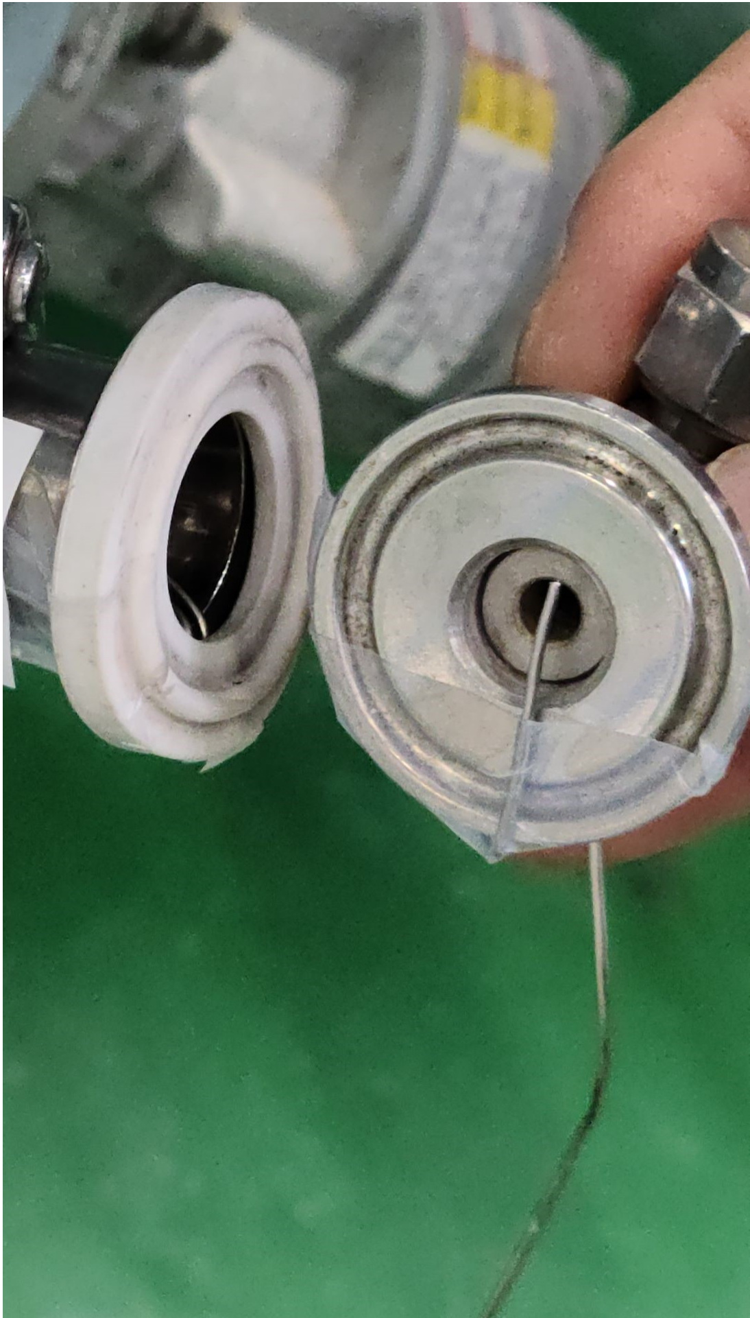
内部温度や内部圧力等を測定する計器（熱電対）を撮影したもの（熱電対は写真右）
